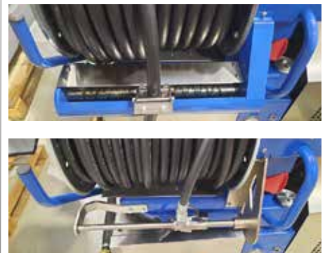
Manual or automatic hose guide Avvolgitubo manuale oppure automatico
